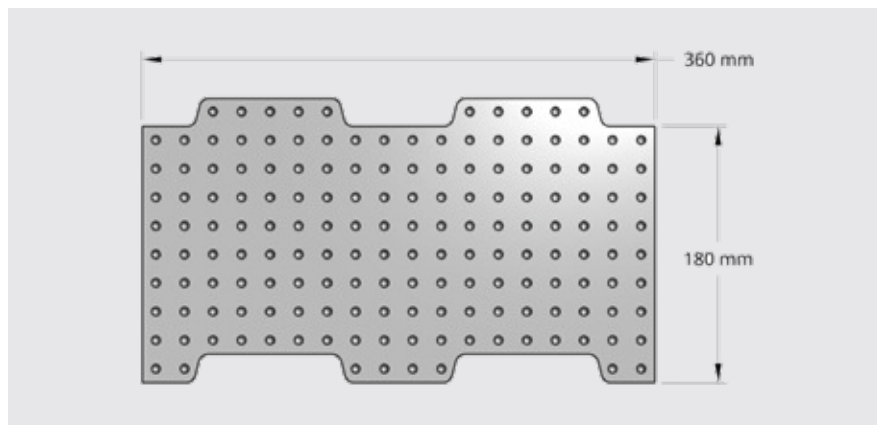
Palette 360×180 Pallet 360×180
