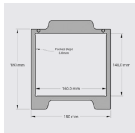
Platte mit quadratischer Ausfräsung Square pocket fixture tray
