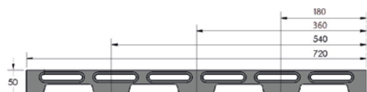
Anschlussleiste 180 / 360 / 540 / 720 Docking rail 180 / 360 / 540 / 720
