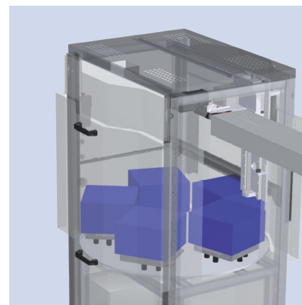
Automatischer Palettenwechsler, 6 Paletten Automatic pallet changer, 6 pallets
